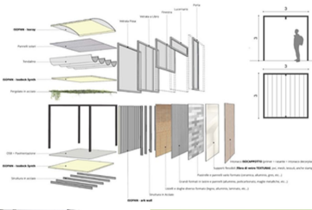
STRUTTURA PERGOLA MODULO VITA
